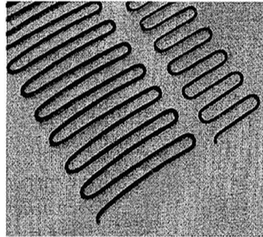
'S'-stirrups
